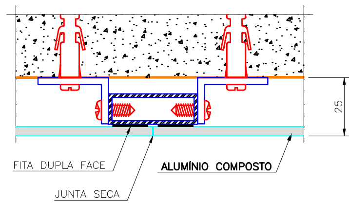
DETALHE TÍPICO DE JUNTA SECA
