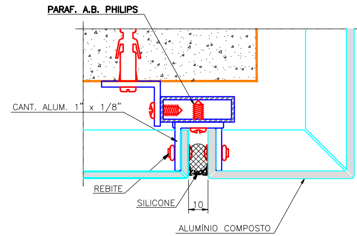
DETALHE DE CANTO
