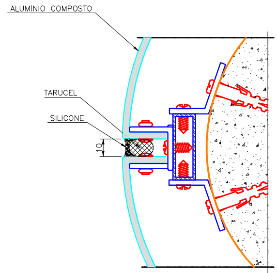
DETALHE DE CHAPA CALANDRADA
