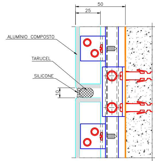
DETALHE TÍPICO DE JUNTA HORIZONTAL
