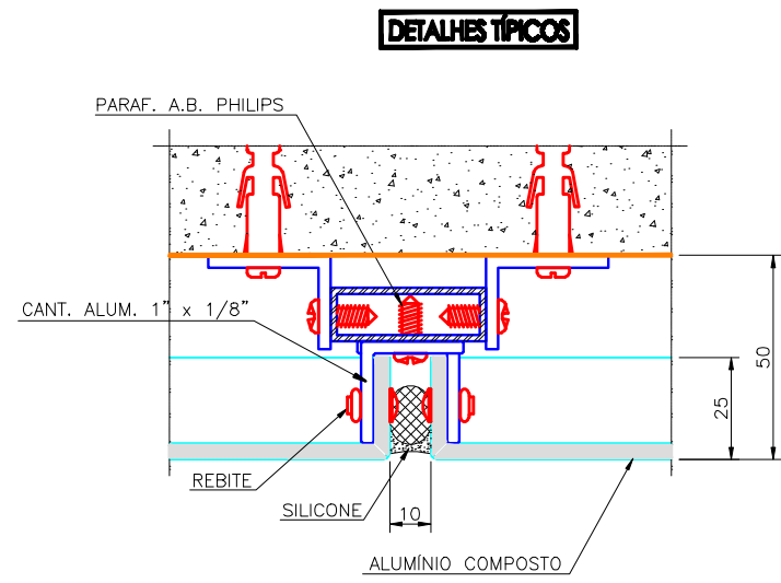
DETALHE TÍPICO DE JUNTA VERTICAL
