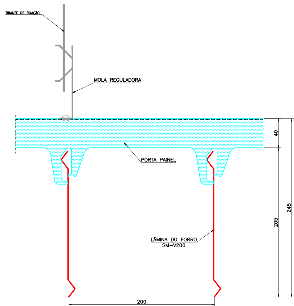
FORRO LINEAR SM-V200 ESCALA: 1:2
