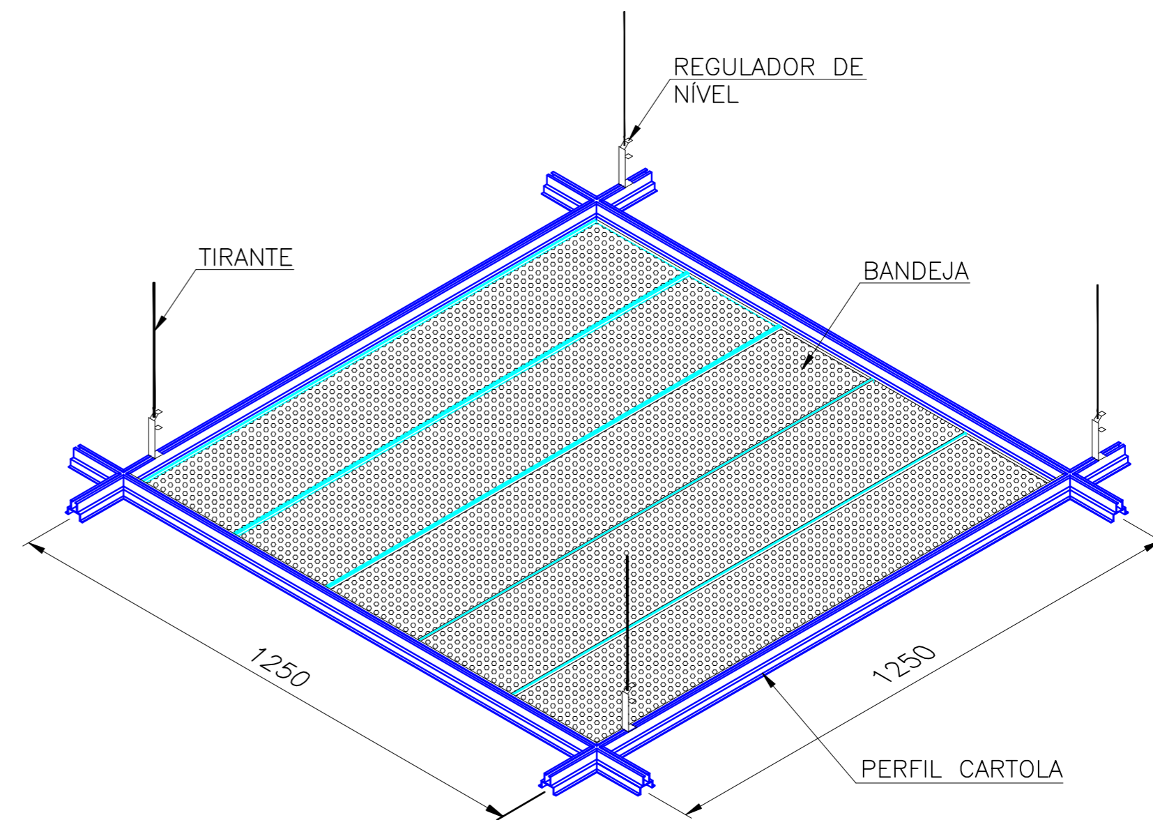
ESQUEMA DE MONTAGEM
