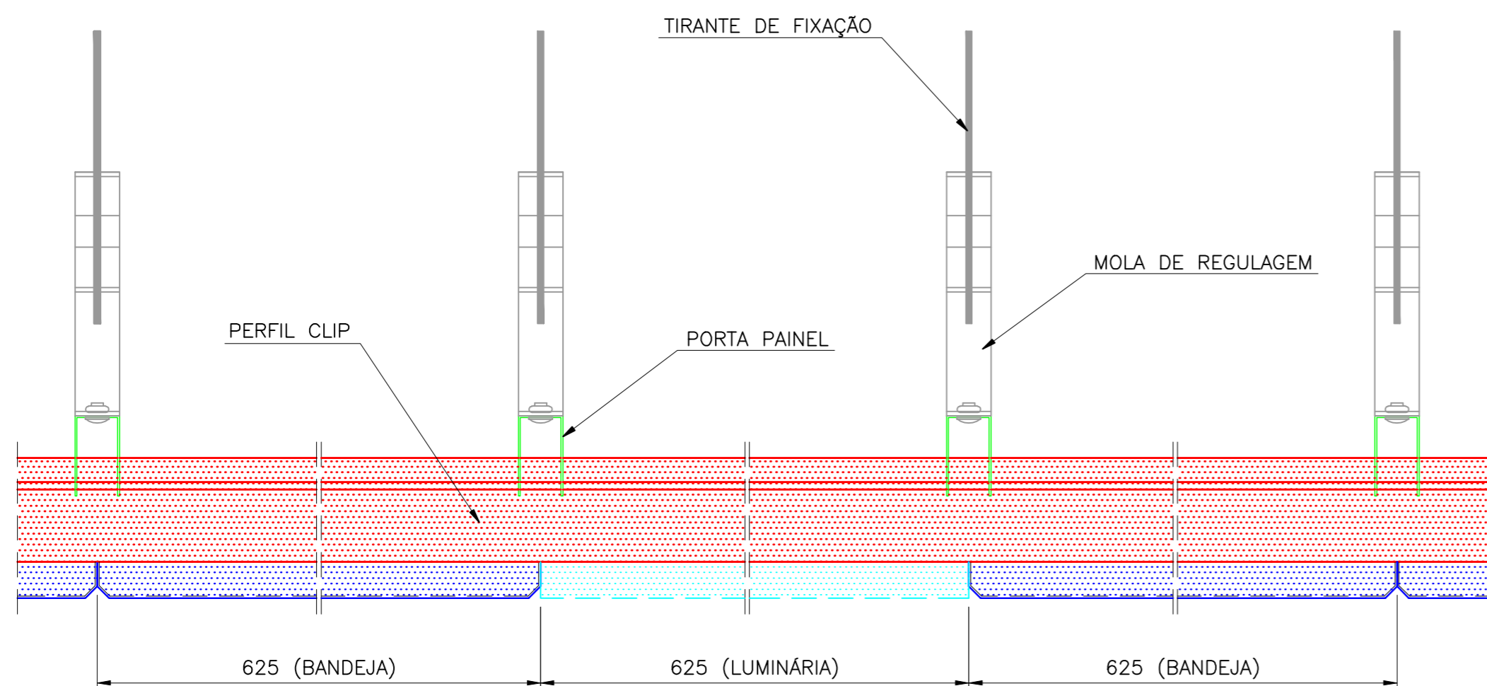
DETALHE DE JUNÇÃO DO FORRO SM-625CI SENTIDO TRANSVERSAL
