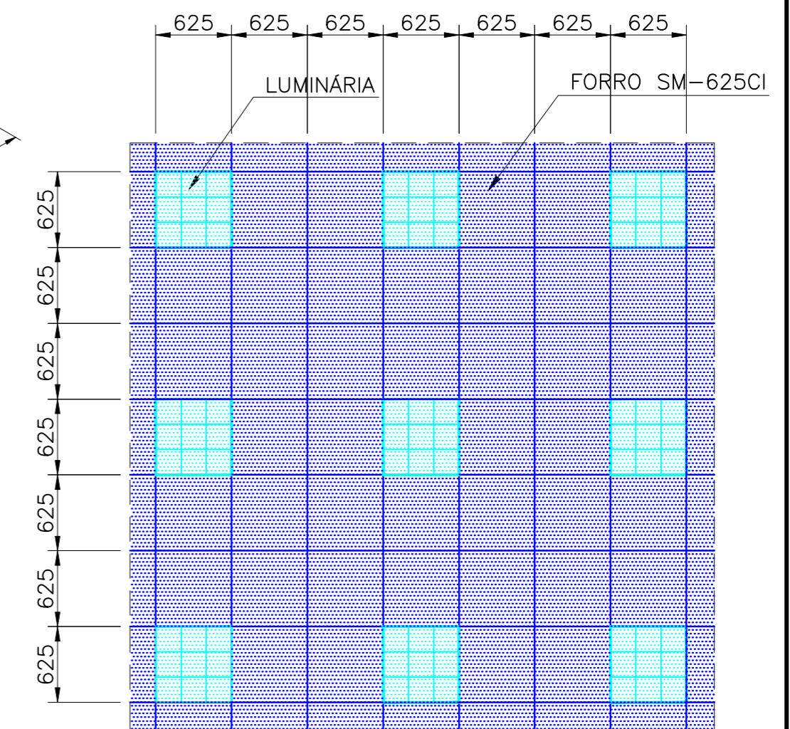
DISTRIBUIÇÃO DO FORRO SM-625CI
