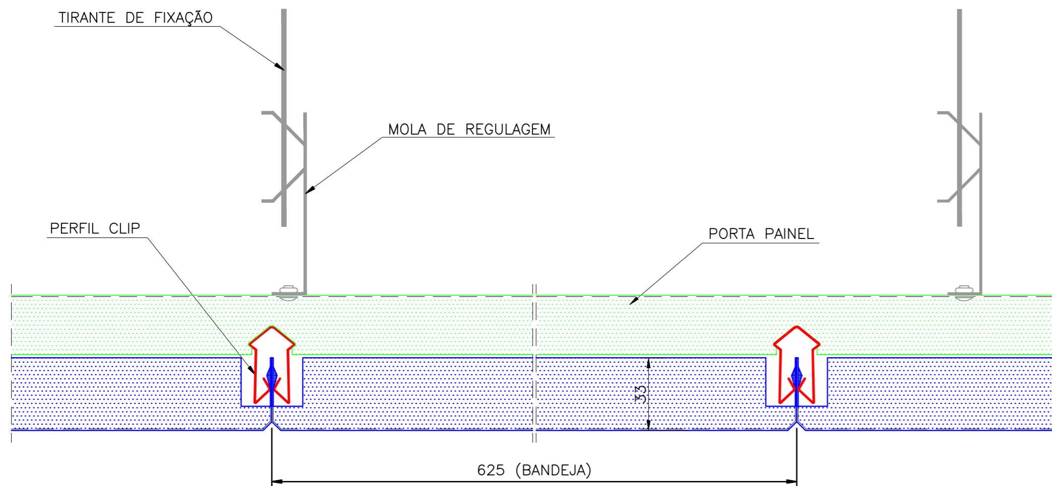
DETALHE DE JUNÇÃO DO FORRO SM-625CI SENTIDO LONGITUDINAL
