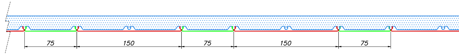
DETALHE DO FORRO SM-150 MESCLADO COM SM-75
