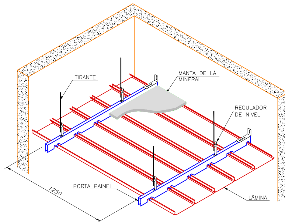
ESQUEMA DE MONTAGEM FORRO SM-150
