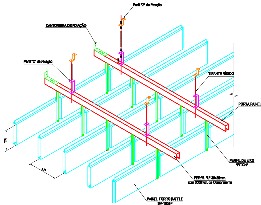
PERSPECTIVA ISOMÉTRICA DO CONJUNTO ESCALA: S/ ESCALA
