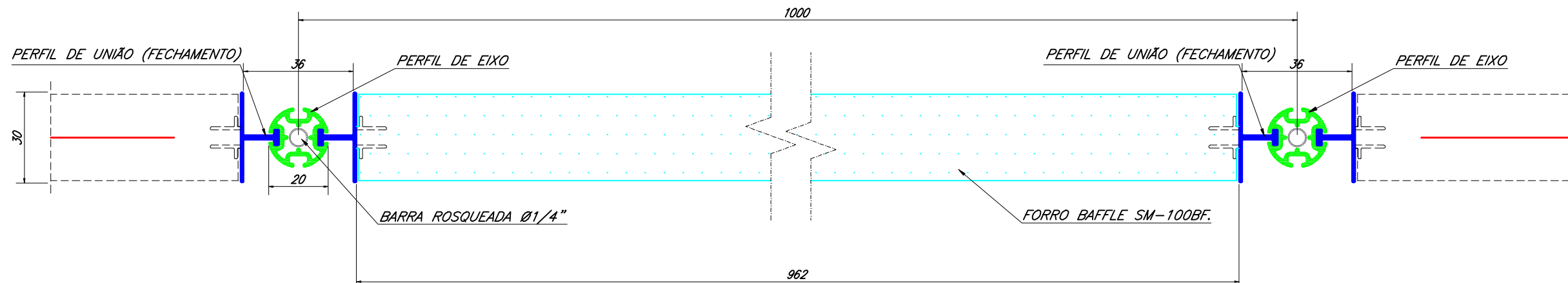
DETALHE DE UNIÃO DOS FORROS ESCALA: 1:1
