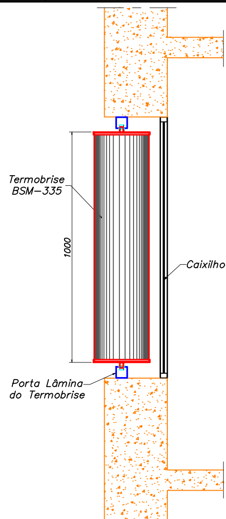
BRISES VERTICAIS DENTRO DO VÃO ESCALA: 1:10
