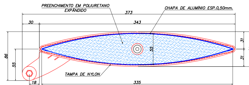
DETALHE DA ASA BRISE BSM-335 Escala: 1:2
