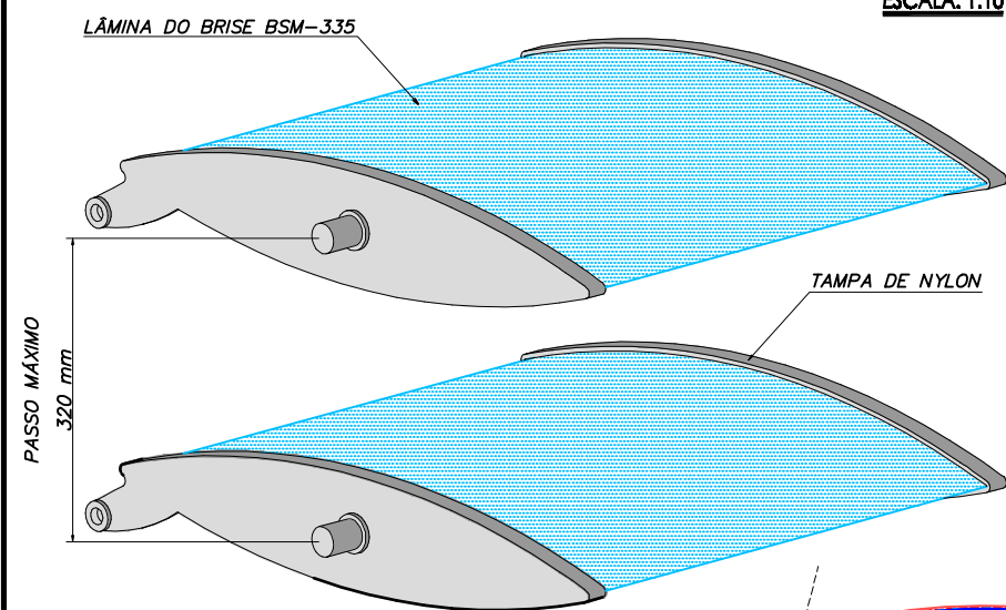
PERSPECTIVA ILUSTRATIVA BSM-335 Escala: 3/4
