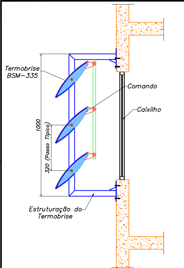
BRISES HORIZONTAIS FORA DO VÃO ESCALA: 1:10
