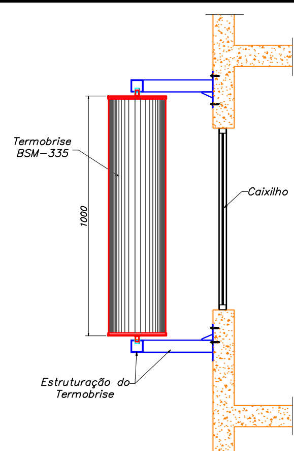
BRISES VERTICAIS FORA DO VÃO ESCALA: 1:10
