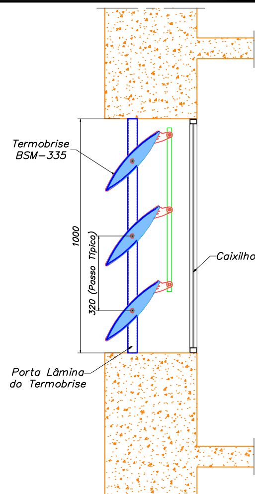
BRISES HORIZONTAIS DENTRO DO VÃO ESCALA: 1:10
