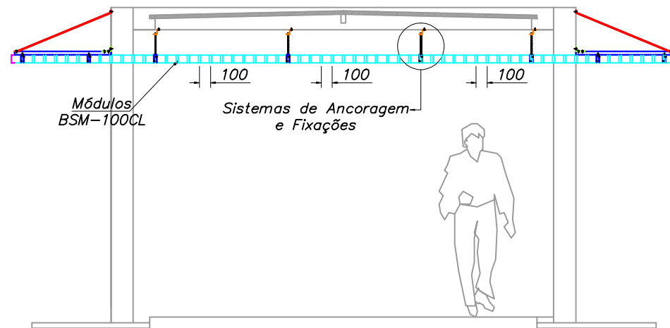
DETALHE DE APLICAÇÃO DO BSM-100CL COMO FORRO Escala: 1:30
