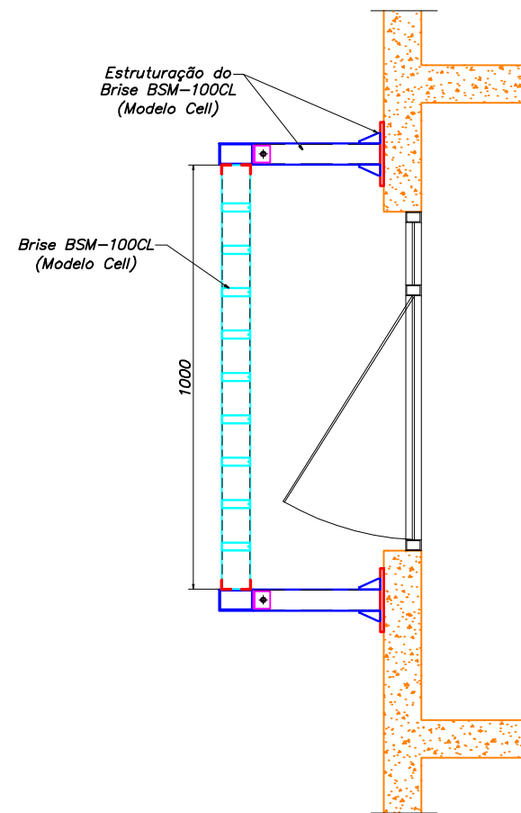
BRISES BSM-100CL FORA DO VÃO ESCALA: 1:10
