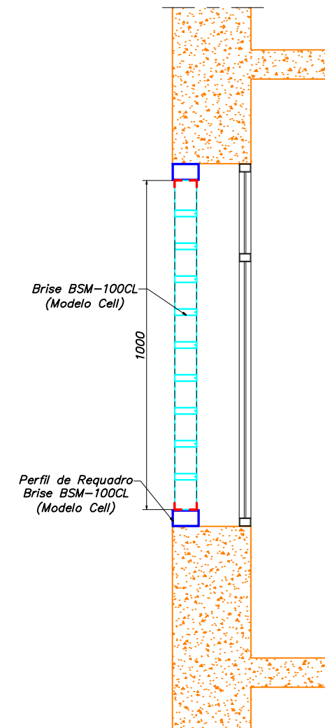
BRISES BSM-100CL DENTRO DO VÃO ESCALA: 1:10
