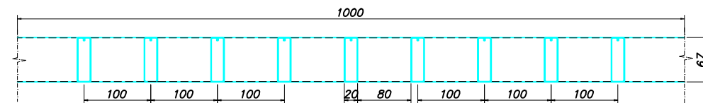
DETALHE DA MALHA DO BRISE BSM-100CL Escala: 1:5
