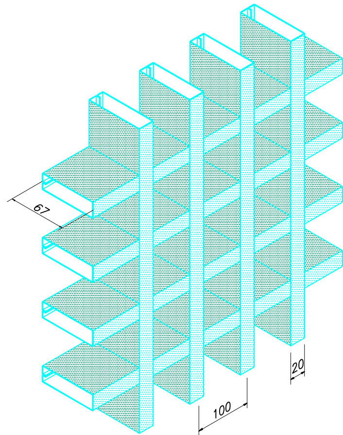
PERSPECTIVA ILUSTRATIVA BSM-100CL Escala: 3/4
