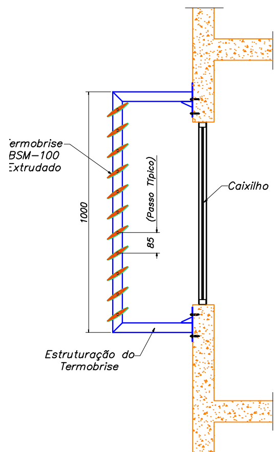
BRISÉS HORIZONTAIS FORA DO VÃO ESCALA: 1:10
