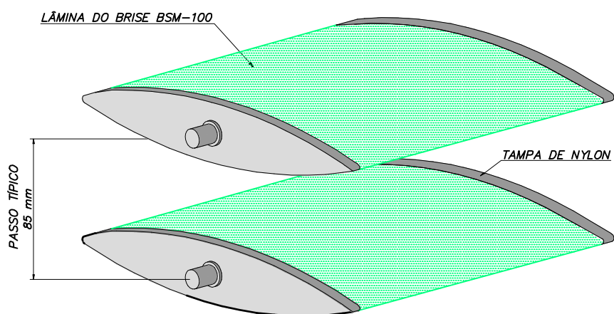
PERSPECTIVA ILUSTRATIVA BSM-100 EXTRUDADO Escala: 3/4
