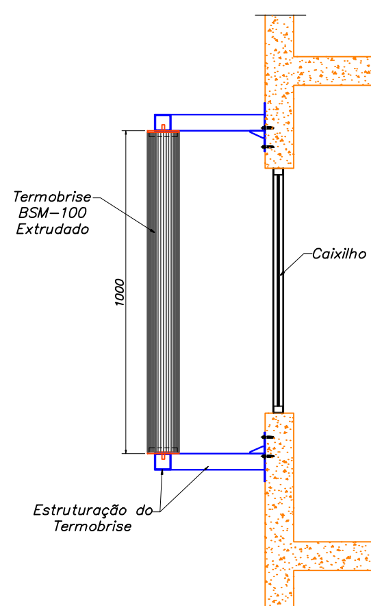
BRISÉS VERTICAIS FORA DO VÃO
