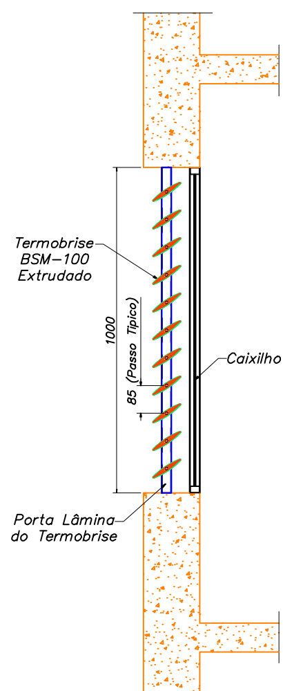
BRISÉS HORIZONTAIS DENTRO DO VÃO ESCALA: 1:10
