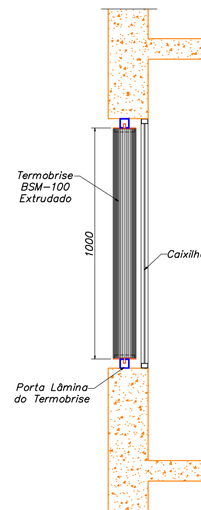
BRISÉS VERTICAIS DENTRO DO VÃO
