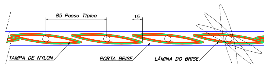
DETALHE DO BRISE SUL METAIS BSM-100 EXTRUDADO Escala: 1:2
